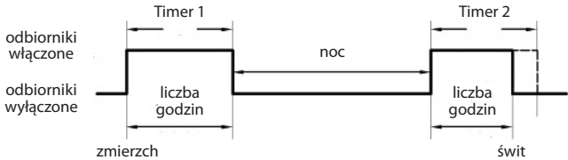
Rys. 4.5 Sposób funkcjonowania systemu dwuzegarowego
