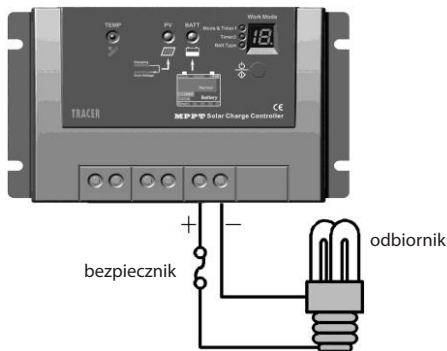
Rys. 3.3 Podłączenie odbiornika
