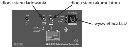
Rys. 4.3 Wskaźniki LED
