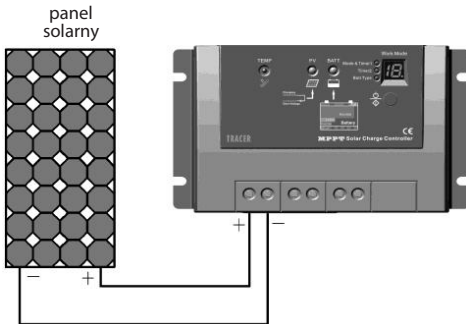
Rys. 3.4 Podłączenie panela solarnego
