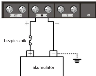
Rys. 3.1 Podłączenie akumulatora
