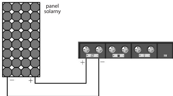
Rys. 3.3 Podłączenie panela solarnego
