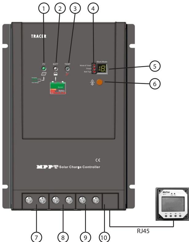
Rys. 2.1 Widok ogólny
